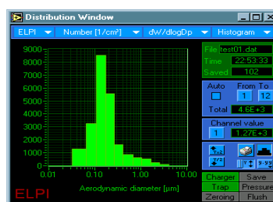
Figure VI-3 : Exemple d'équipement de classification par inertie et détection électrostatique : ELPI. Type d'histogramme obtenu, exprimé en concentration particulaire.
