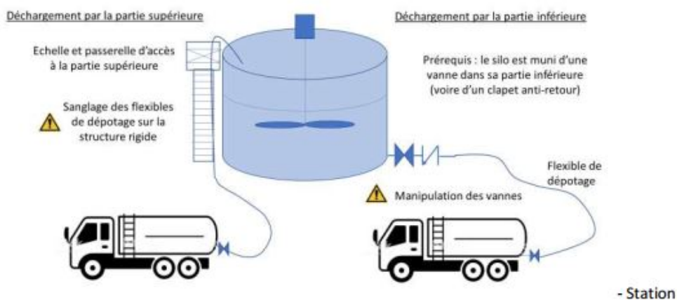
Alternatives en cas d'absence de tuyauterie de dépotage rigide
