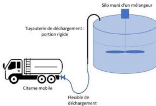
Déchargement de lait de chaux dans un silo de stockage liquide
